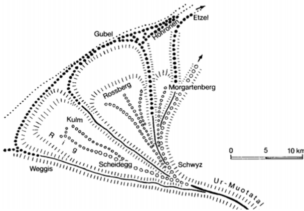
Fächer der Rigi-Rosserg-Schüttung (aus VOGEL und HANTKE, 1988).
